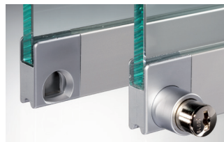
El uñero integrado en la casaca, el cerradero y la cerradura armonizan en las medidas y el diseño con los perfiles de la casaca.
