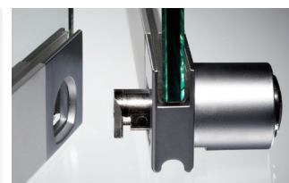
En el mecanismo patentado de pestillo de seguridad Secura, un bulón en forma de L integrado en la hoja delantera se encaja en el cerradero de la hoja posterior, evitando así la separación forzosa de las dos hojas. (A)
