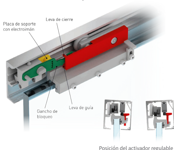
Cerradura eléctrica para Portavant M50 y M80
