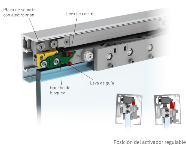
Cerradura eléctrica para Portavant G120
