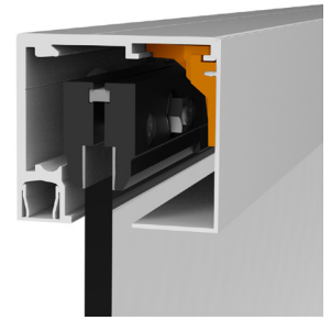
Clip para tapeta con geometría pensada para reforzar la rigidez de la tapeta.
