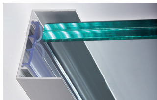
El perfil de marco Robustus permite montar al ras la hoja y el perfil de la casaca, visualizando así una imagen de gran atractivo.
